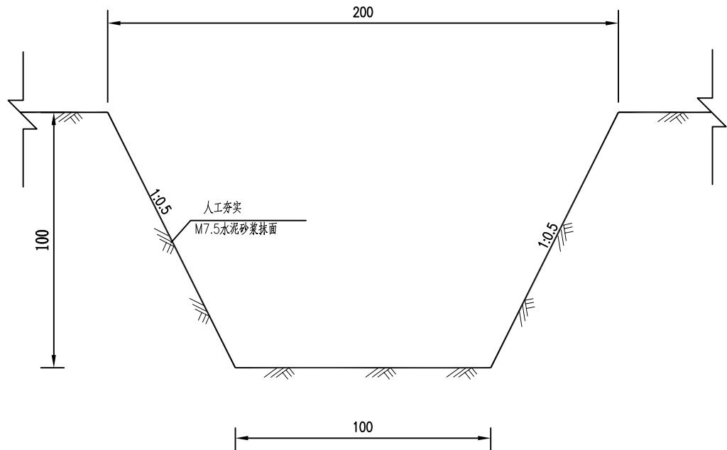
临时沉砂池A-A剖面图 1:20
