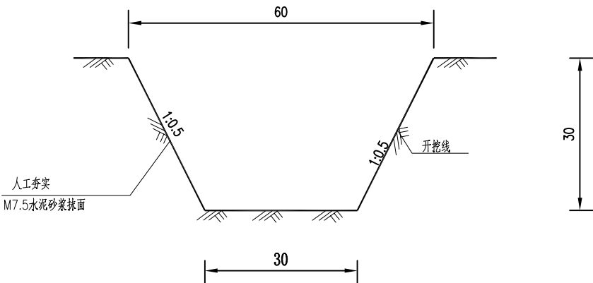
临时排水沟典型断面图 1:10
