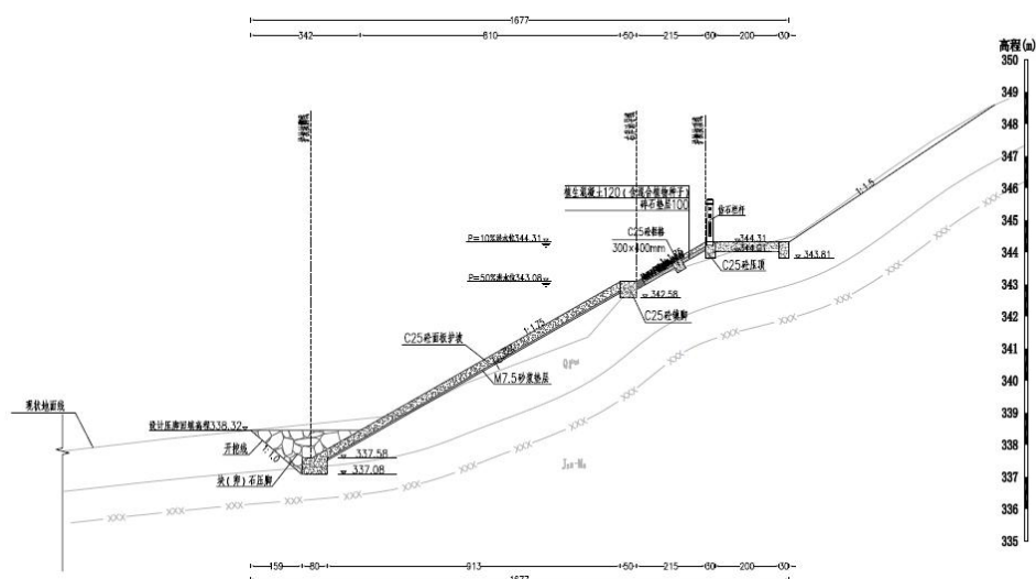
图 2-10 御临河川主乡段护岸 YLK23+147 典型断面图
