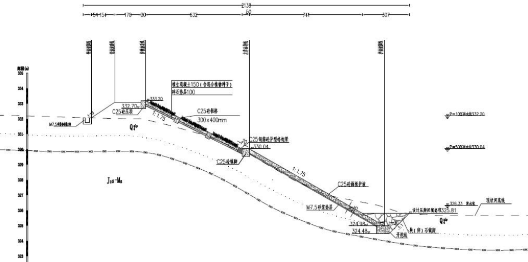
图 2-11 御临河高穴镇段堤防 YLK30+563 典型断面图
