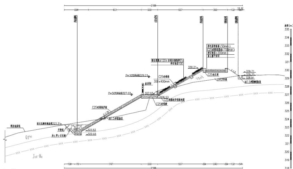
图 2-18 御临河妈妈镇段堤防 YLK37+900 断面图
