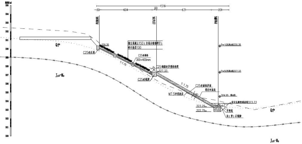
图 2-15 御临河高穴段护岸防 YLK34+775 典型断面图
