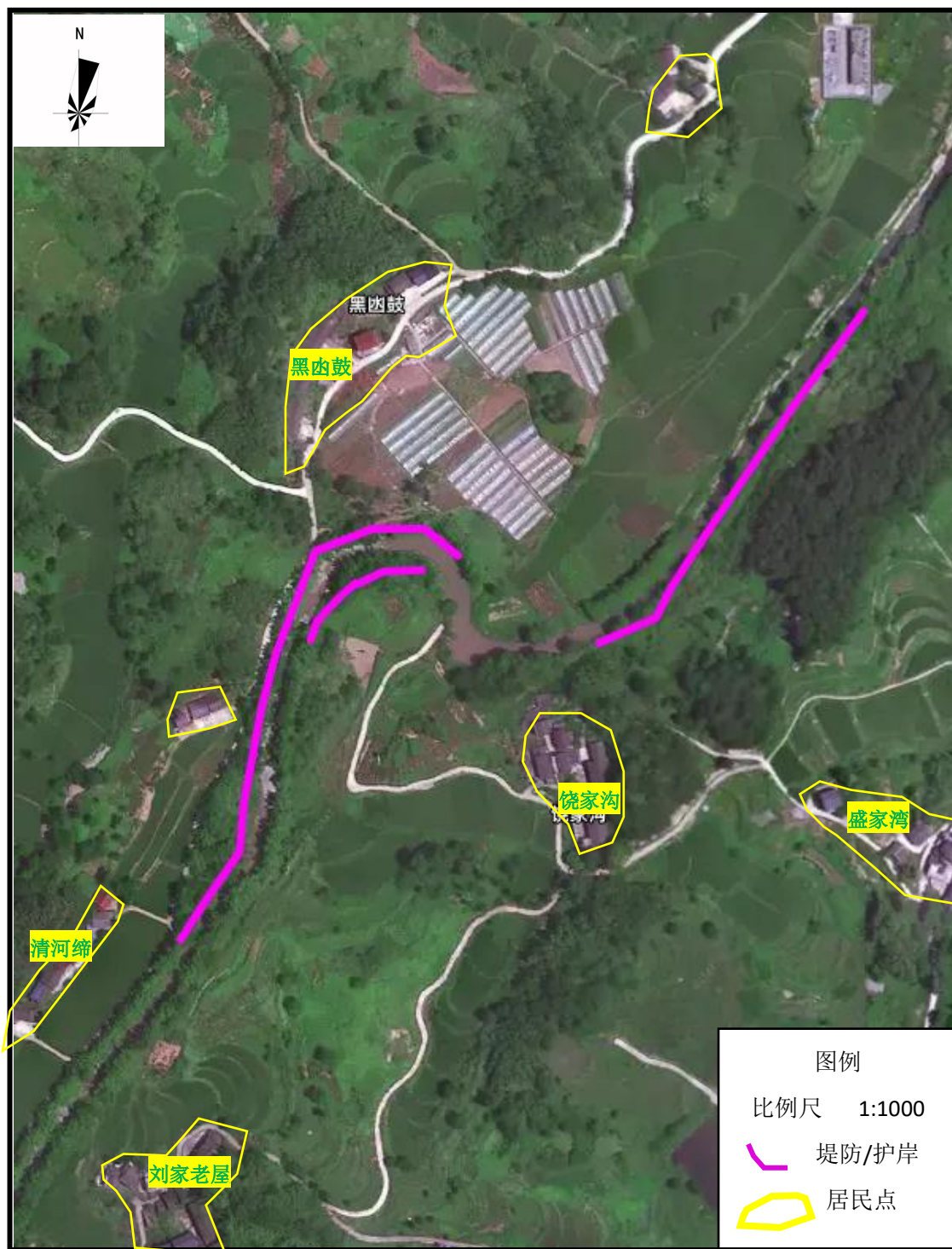
附图 4-2 团坝镇 2 段外环境关系图
