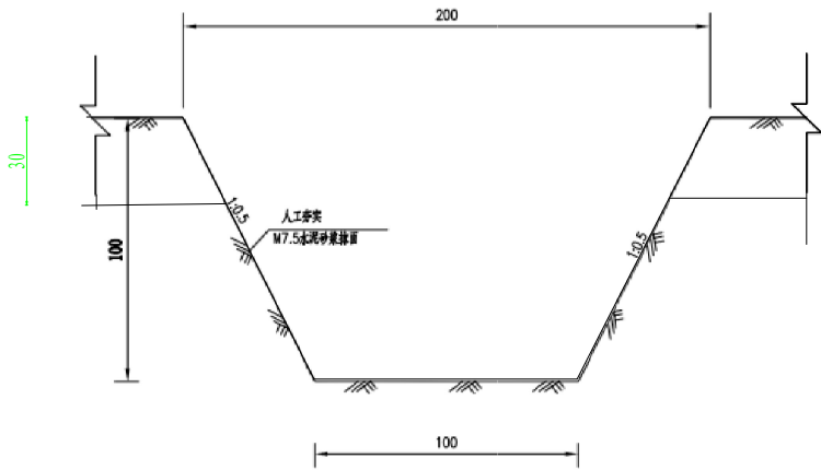
临时沉砂池A-A剖面图
