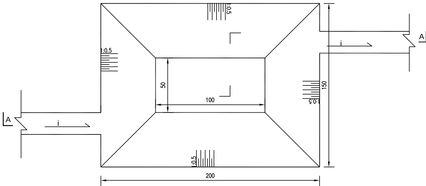
临时沉砂池典型平面图 1:20
