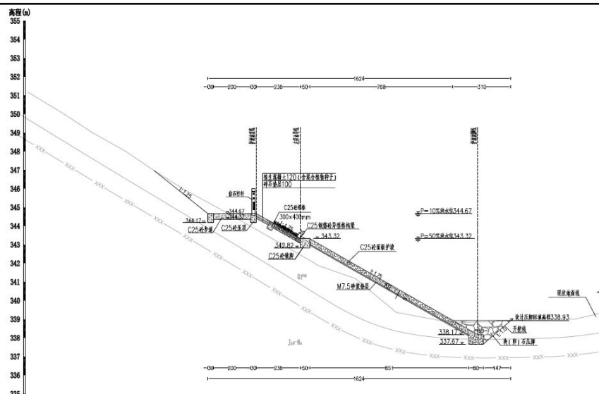
图 2-9 御临河川主乡段护岸 YLK21+590 断面图
