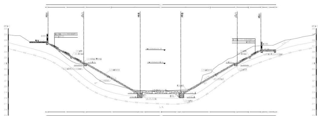
图 2-23 御临河妈妈镇段护岸 YLK40+325 断面图
