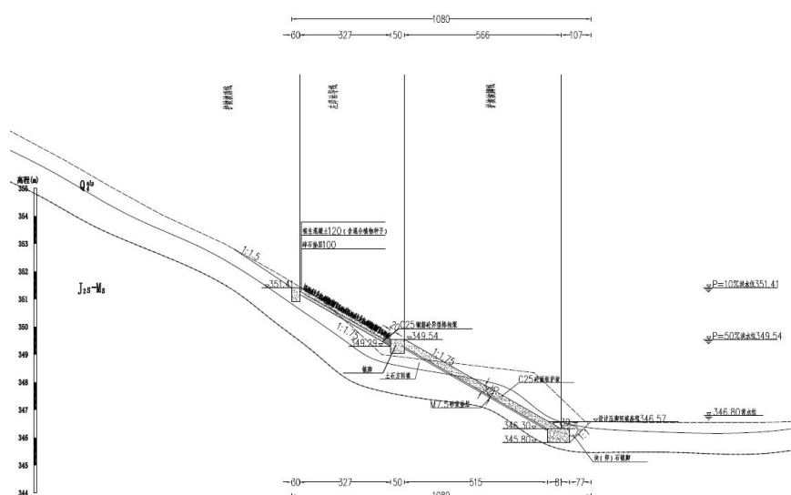
图 2-6 御临河团坝镇段护岸 YLK12+980 典型断面图
