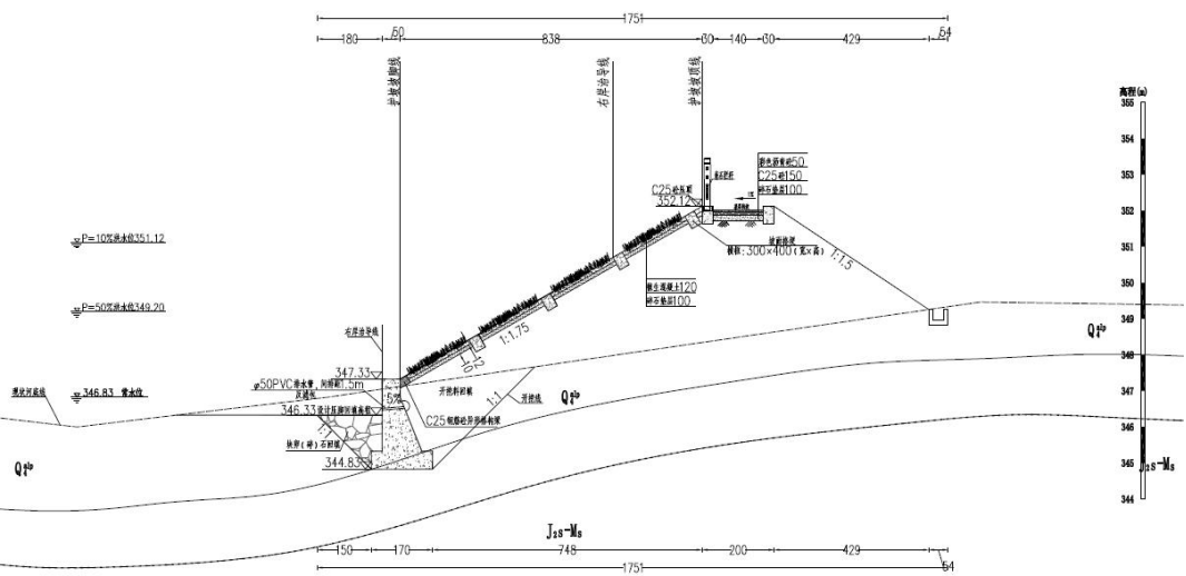
图 2-1 御临河团坝镇段堤防 YLK13+186 典型断面图
