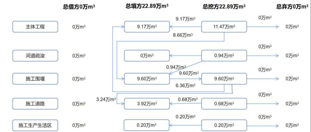
图 2-24 御临河大竹段防洪除涝工程（一期）土石方平衡图
