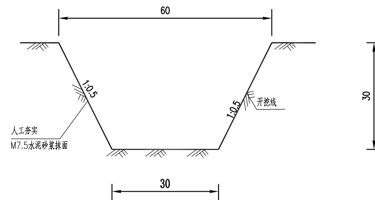
排水土沟典型断面图
