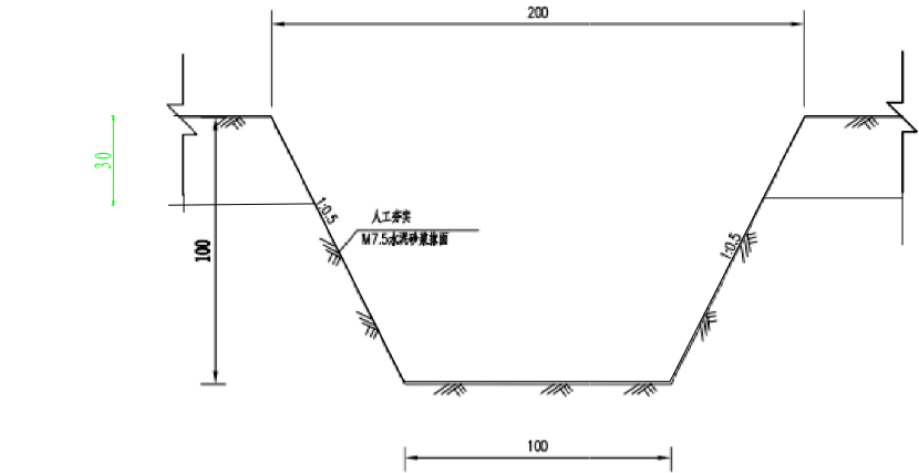
临时沉砂池A-A剖面图
