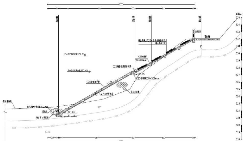
图 2-20 御临河妈妈镇段护岸 YLK36+700 典型断面图
