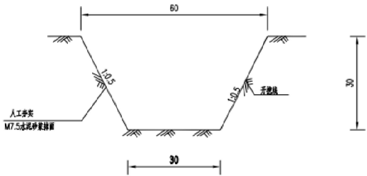
临时排水沟典型断面图
