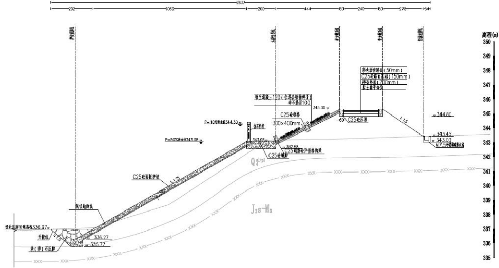
图 2-8 御临河川主乡段堤防 YLK23+273 断面图
