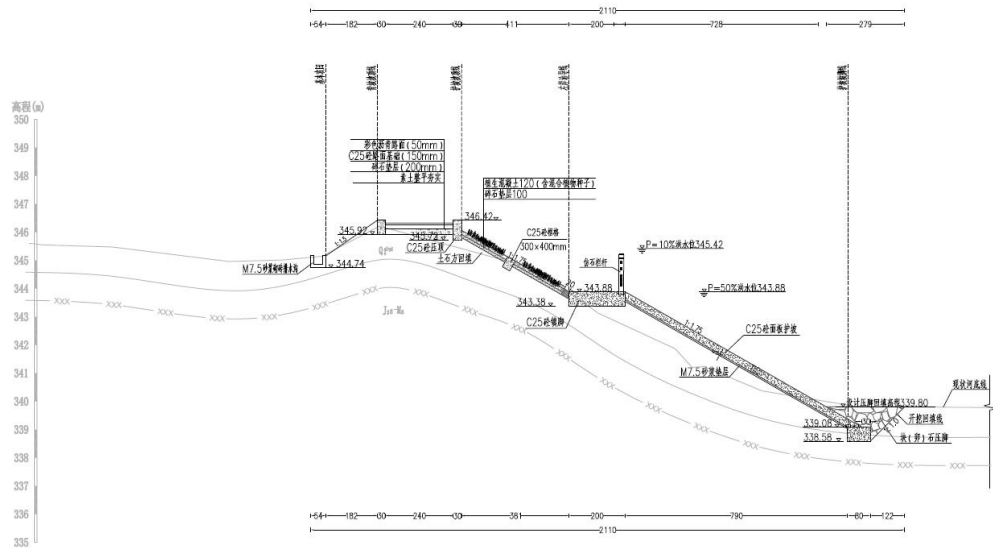
图 2-7 御临河川主乡段堤防 YLK19+367 断面图
