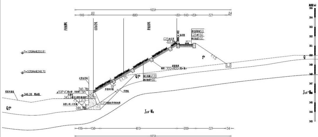
图 2-2 御临河团坝镇段堤防 YLK13+522 典型断面图
