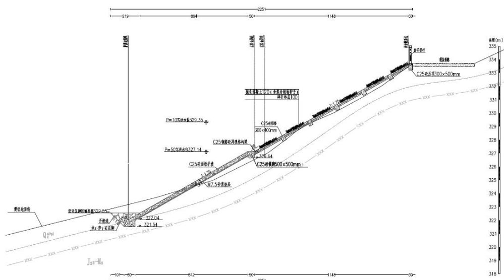
图 2-21 御临河妈妈镇段护岸 YLK37+460 典型断面图
