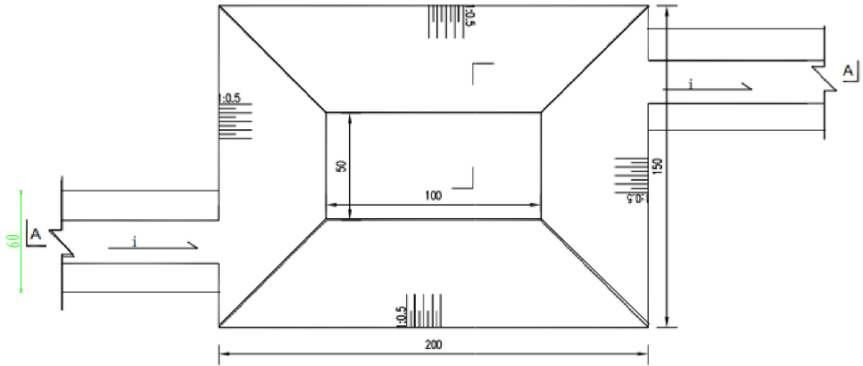
临时沉砂池典型平面图
