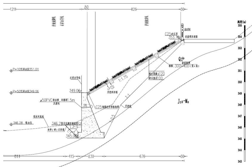
图 2-5 御临河团坝镇段护岸 YLK13+277 典型断面图
