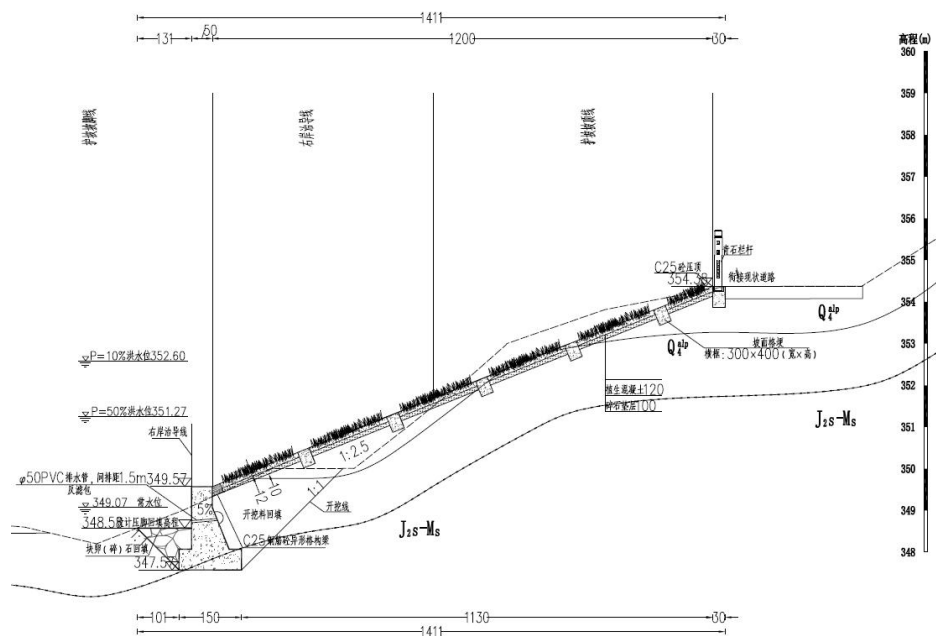
图 2-4 御临河团坝镇段护岸 YLK12+267 典型断面图
