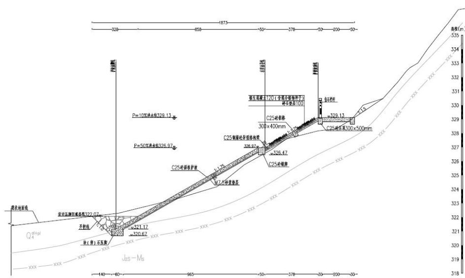
图 2-22 御临河妈妈镇段护岸 YLK38+100 典型断面图
