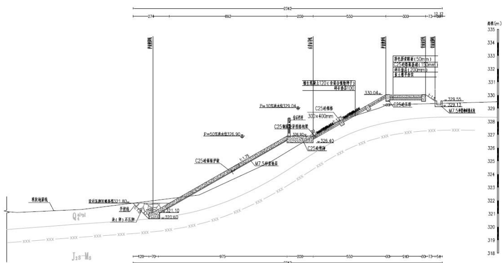
图 2-19 御临河妈妈镇段堤防 YLK38+689 断面图
