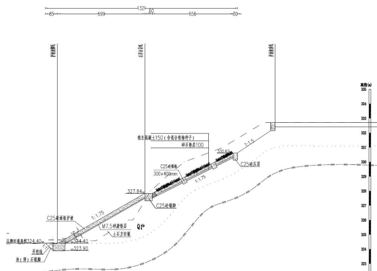
图 2-16 御临河高穴段护岸 YLK33+975 典型断面图
