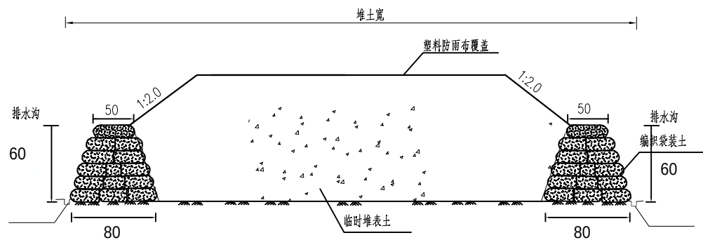
A-A剖面图
